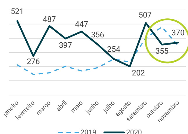
Importação de Inversores 2019 e 2020 [MW]
