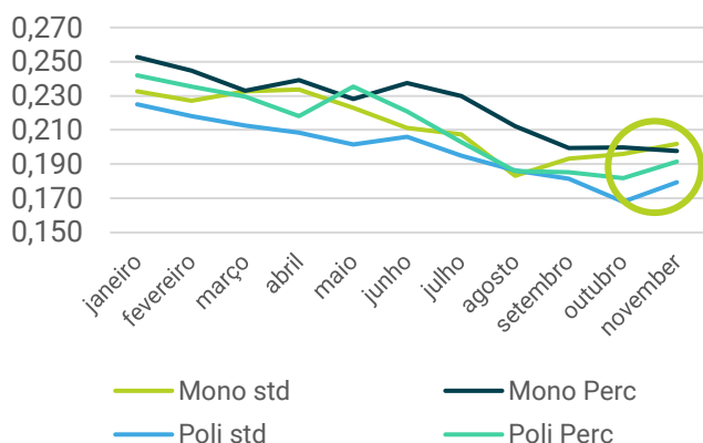
Preço FOB [US$/Wp]
